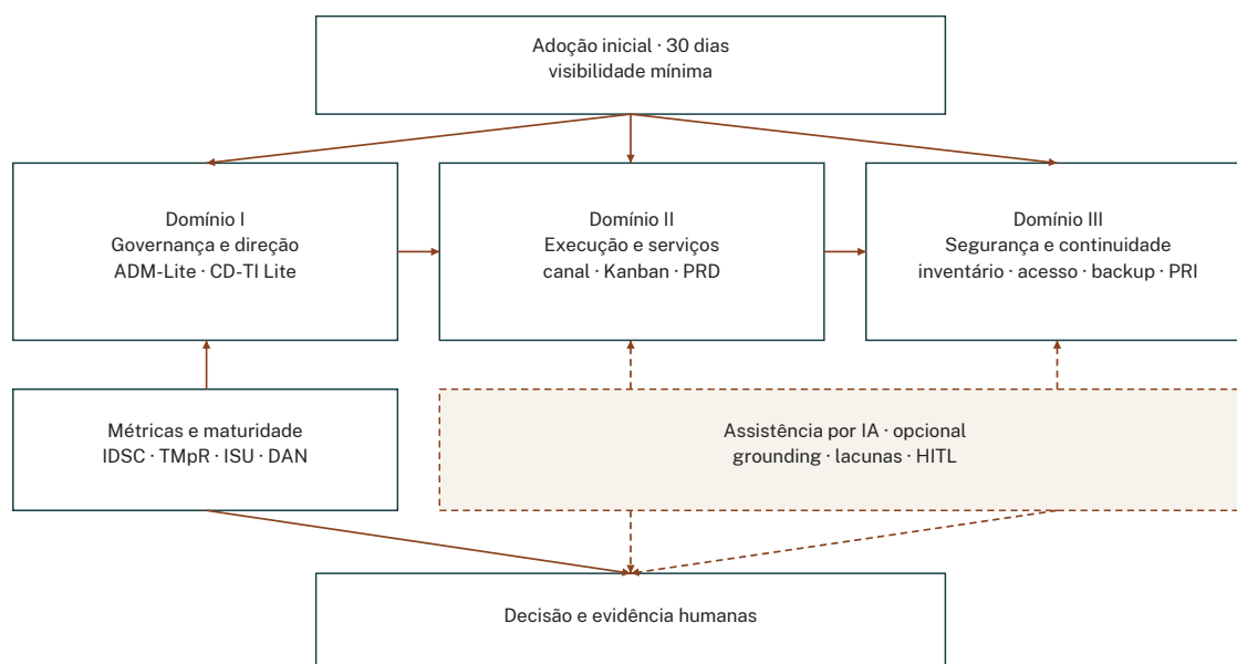
Figura 2: Arquitetura conceitual do GEAR. As setas representam ciclos de informação e decisão, não uma sequência rígida.
